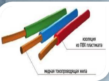
Монтажні провода
